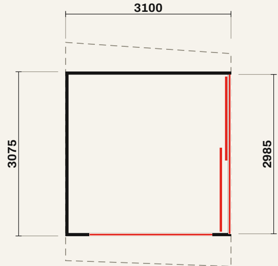
FLOOR PLAN · MM
